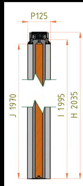
Vertikální řez pouzdrum ABSOLUTE LINE Komfort
